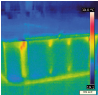
Wärmeverlustprüfung mit dem Nordic Insulation System
